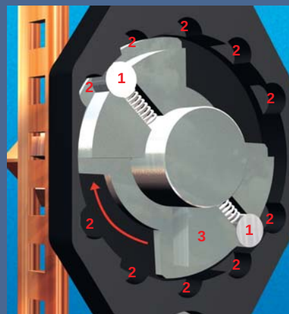
W miarę dalszego przekręcania klamki, wałki ryglujące (1) zabierane są przez obracane sprzęgło (3), aż do ponownego umieszczenia ich w kolejnych otworach(2).
