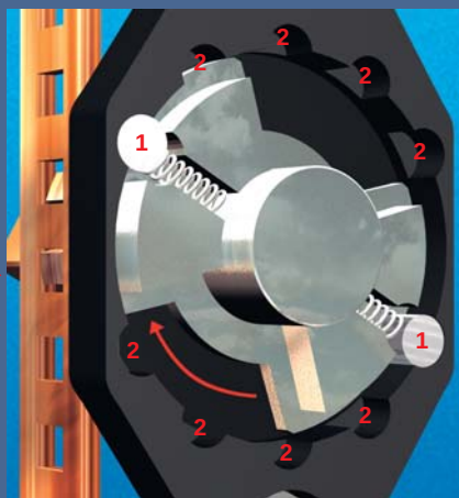
Przekręcenie klamki okiennej powoduje przesuwanie przy towarzyszącym temu precyzyjnym dźwiękowi, wałków ryglujących (1) dociskanych sprężynkami, aż do umieszczenia ich w otworach znajdujących się na obwodzie obudowy (2) – w ten sposób powstaje typowe klikanie dla klamki Secustik® – z dodatkowym słyszalnym akcentem bezpieczeństwa!
