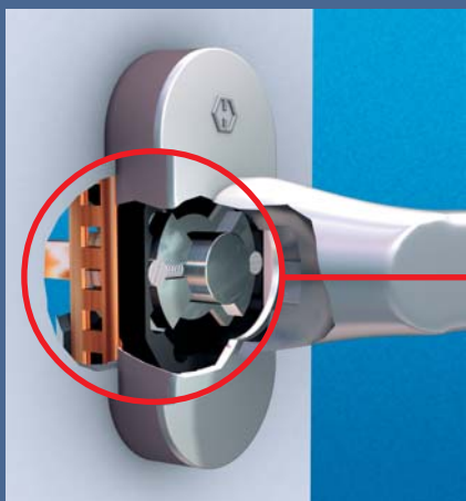
Opatentowany mechanizm blokujący klamki okiennej Secustik®
